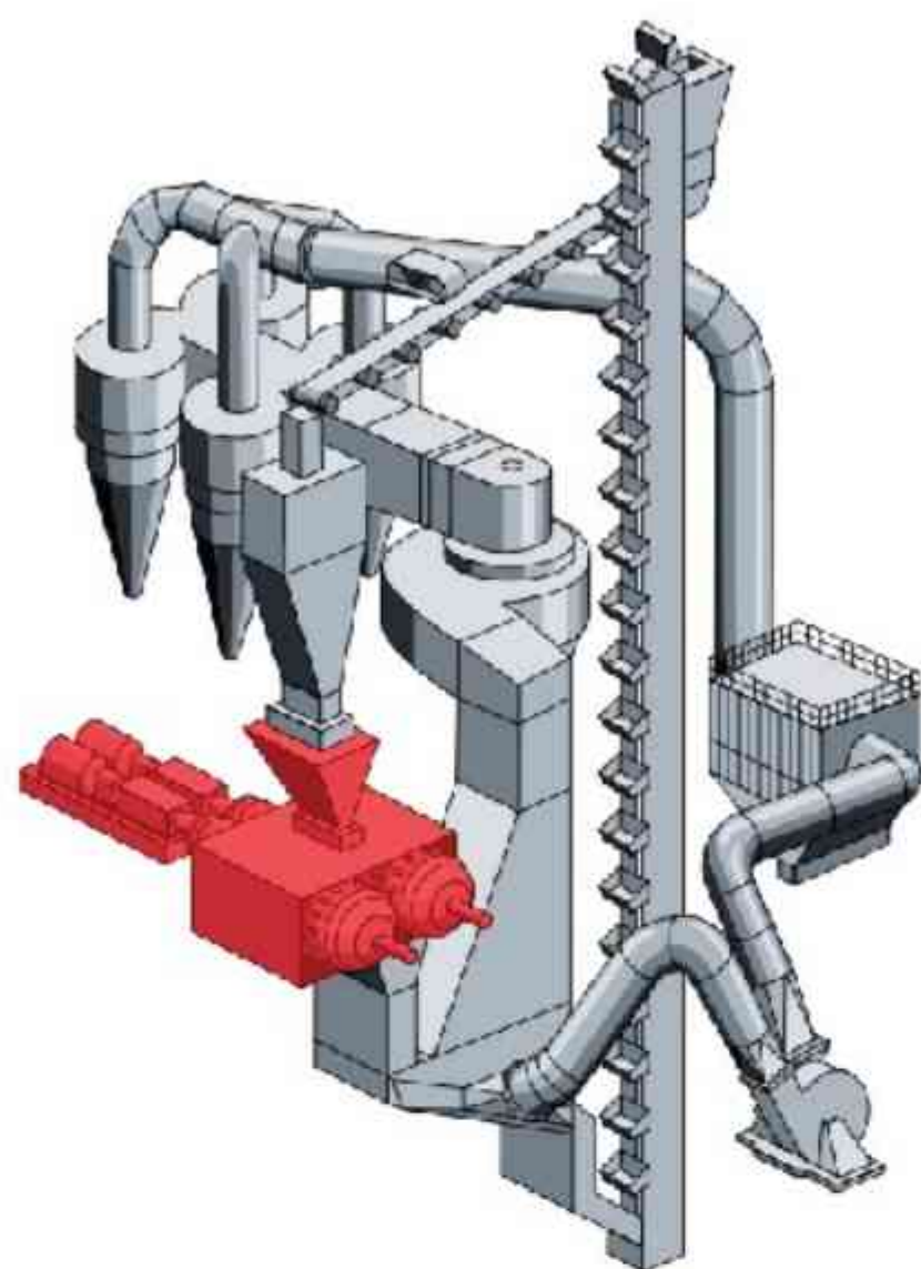
Roller Press
